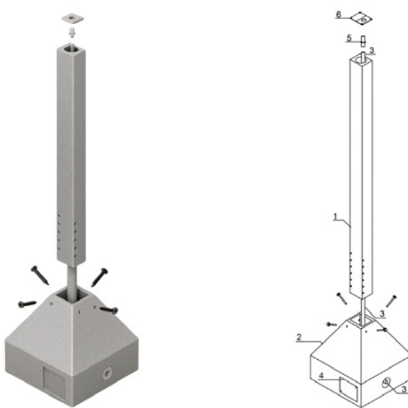
Diseño de poste modular desarrollado y patentado por Uniguajira
